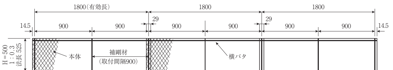
正面図
