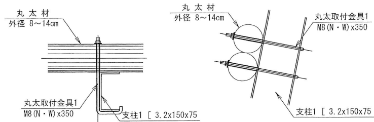
丸太材取付部 詳細図 S=1:5
