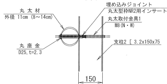
丸太材取付部 詳細図 S=1:5
