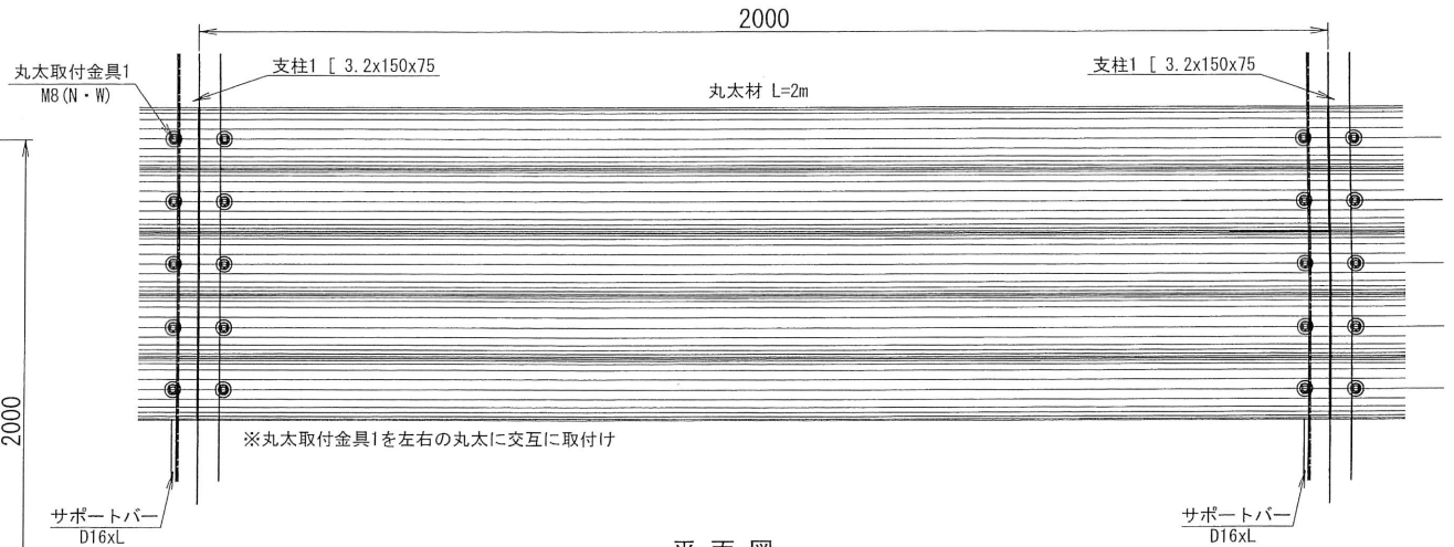
平面図 S=1:5
