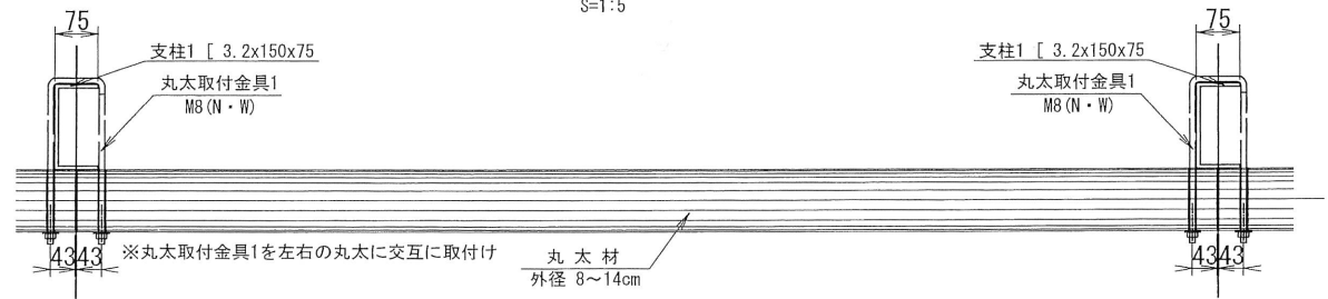
平面図 S=1:5
