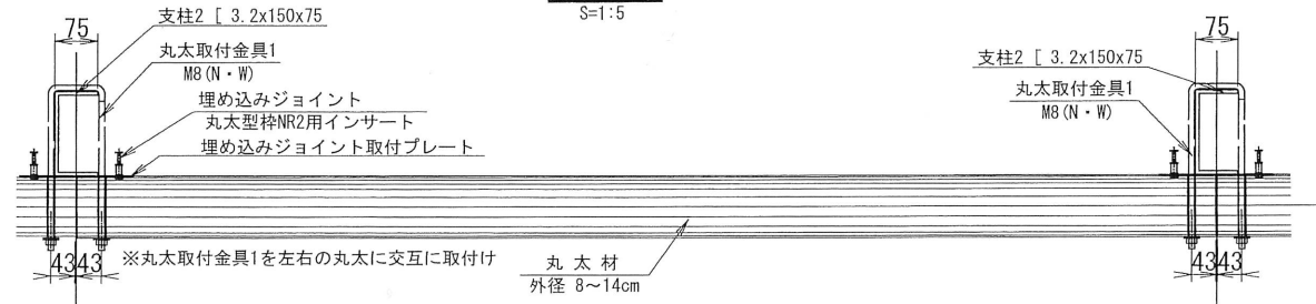
埋め込みジョイント 取付けプレート詳細図 S=1:5
