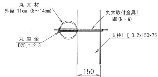
丸太材取付部 詳細図 S=1:5
