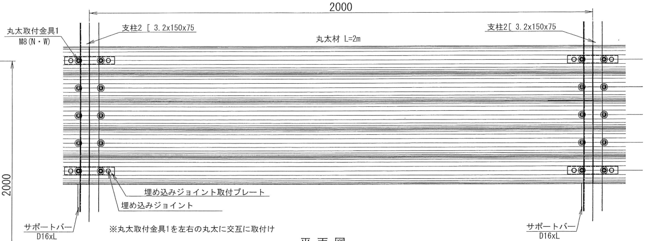
平面図 S=1:5
