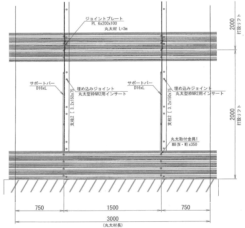
正面図 S=1:10
