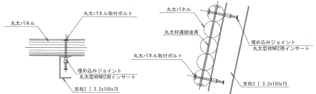
丸太パネル取付部 詳細図 S=1:5
