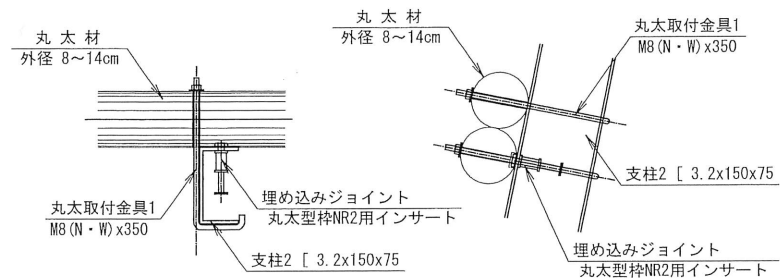
丸太材取付部 詳細図 S=1:5
